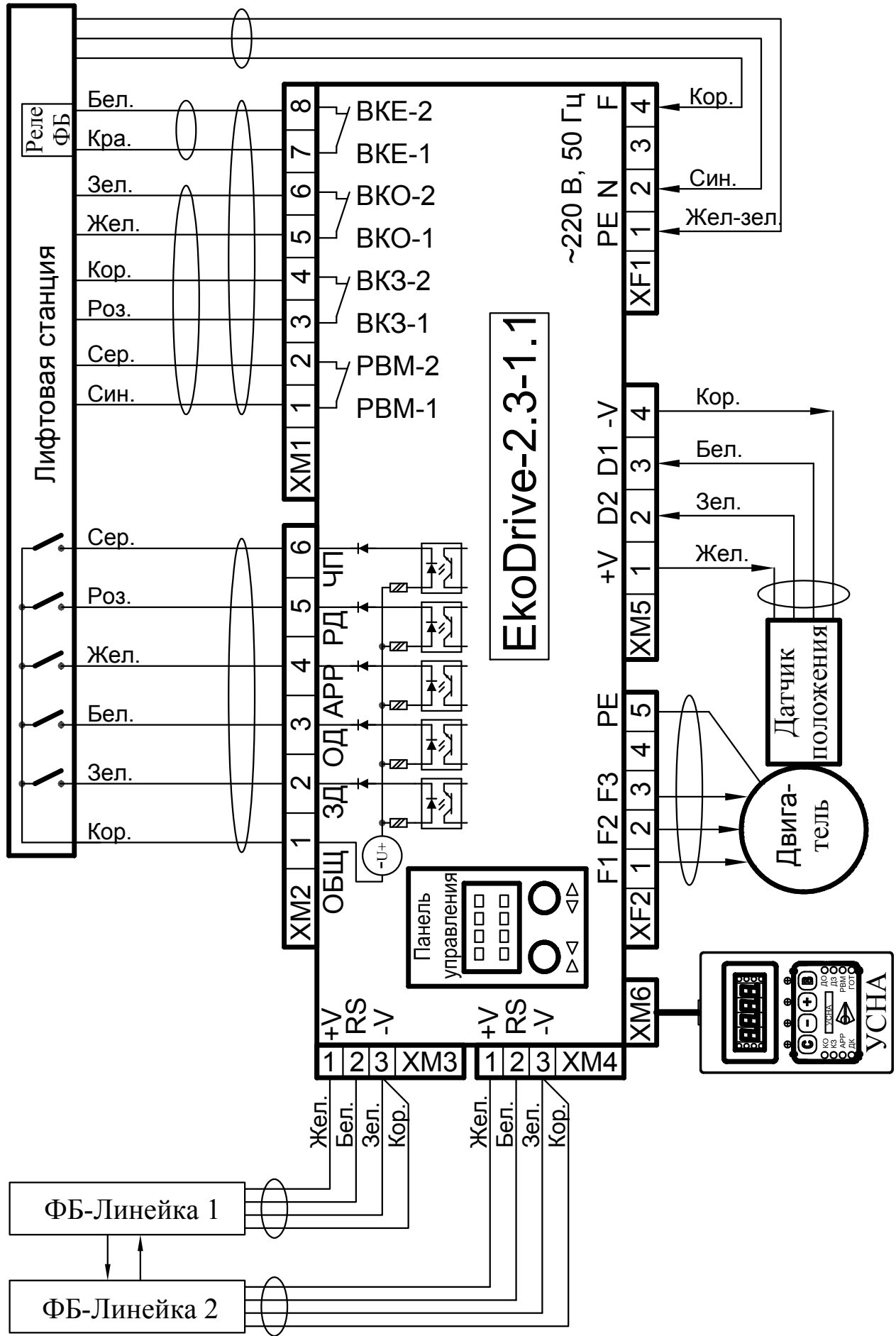
Рис 2. Блок-схема подключения фотоборьера ФБ-1.0-П.1.0 к Экодрайв и лифтовой станции.
