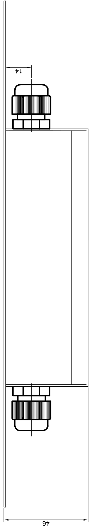
Рис 3. Габаритные размеры Контроллера ФБ-014.1-КО
