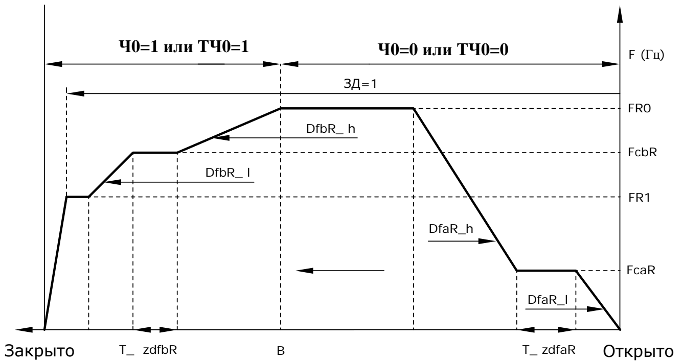
Рис. 9. Диаграмма закрытия по таблице 3 для лифтовых дверей.
